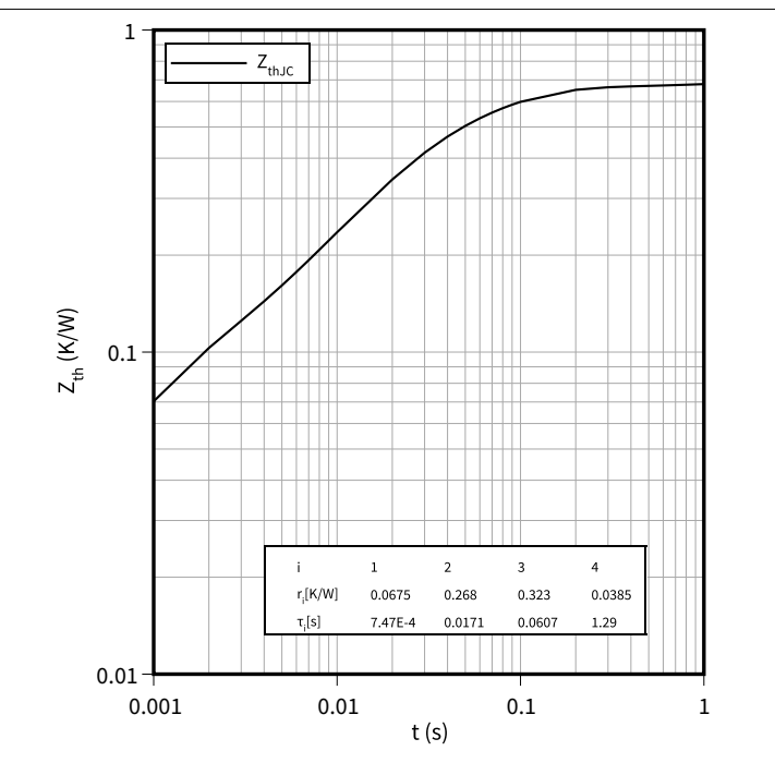
瞬态热阻抗, 二极管,整流器 Z_{th} = f(t)
