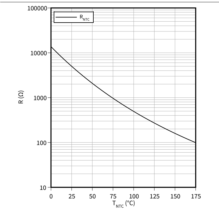
温度特性, 负温度系数热敏电阻 R = f(T_{NTC})
