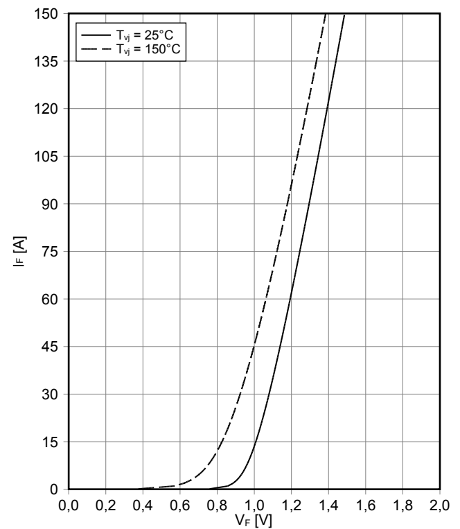
正向偏压特性 二极管,整流器 (典型) forward characteristic of Diode, Rectifier (typical) I_F = f(V_F)
