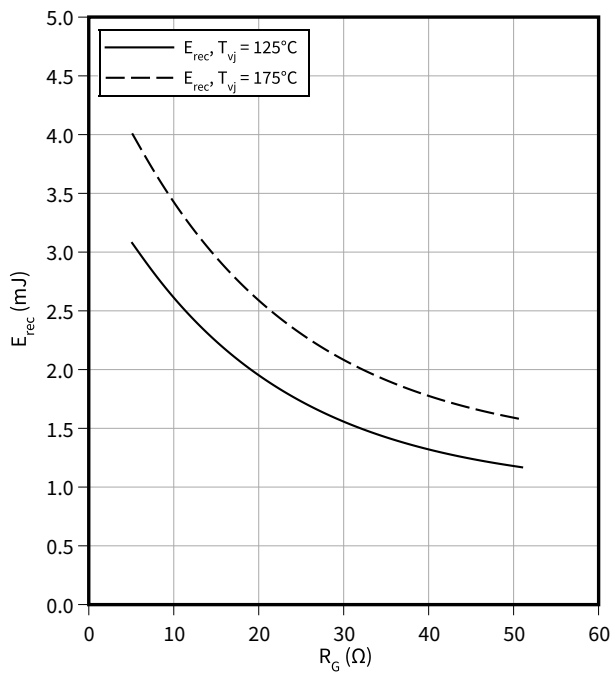
スイッチング損失 (typical), Diode、インバータ E_{rec} = f(R_G) I_F = 50 A, V_{CC} = 600 V
