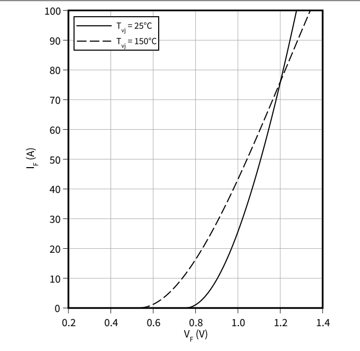
正向特性 (典型), 二极管, 制动-斩波器
