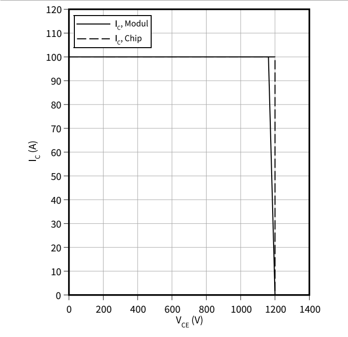
逆バイアス安全動作領域 (RBSOA), IGBT- インバータ I_C = f(V_{CE}) R_{Goff} = 5.1 \Omega , V_{GE} = \pm 15 \text{ V} , T_{vj} = 175 \text{ °C}
