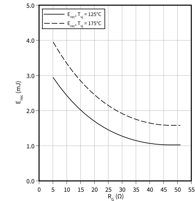
开关损耗（典型), 二极管,逆变器 E_{rec} = f(R_G) I_F = 50 A, V_{CC} = 600 V
