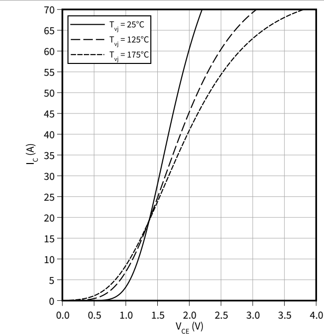
输出特性（典型）, IGBT, 制动-斩波器 I_C = f(V_{CE}) V_{GE} = 15\text{ V}
