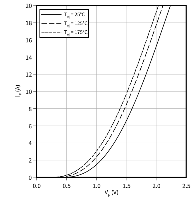
正向特性（典型）, 二极管, 制动-斩波器 I_F = f(V_F)
