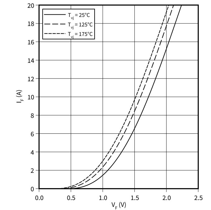
Durchlasskennlinie der (typisch), Diode, Chopper I_F = f(V_F)
