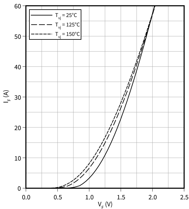
正向特性（典型）, 二极管, D13-D18
