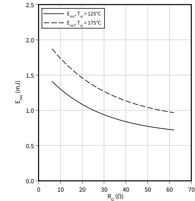
开关损耗（典型），二极管,逆变器 E_{rec} = f(R_G) I_F = 25 A, V_{CC} = 600 V
