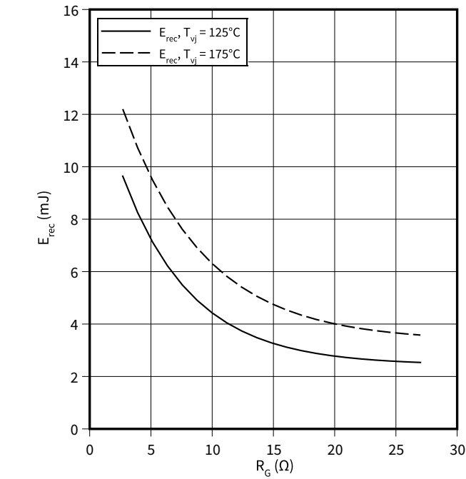
开关损耗（典型），二极管，逆变器 E_{rec} = f(R_G) I_F = 200 A, V_{CC} = 600 V
