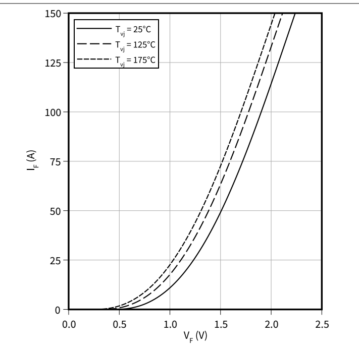
正向特性 (典型), 二极管, 制动-斩波器 I_F = f(V_F)
