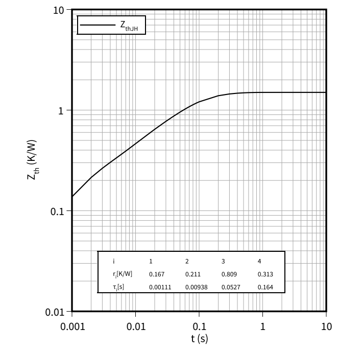
過渡熱インピーダンス, Diode、整流器 Z_{th} = f(t)
