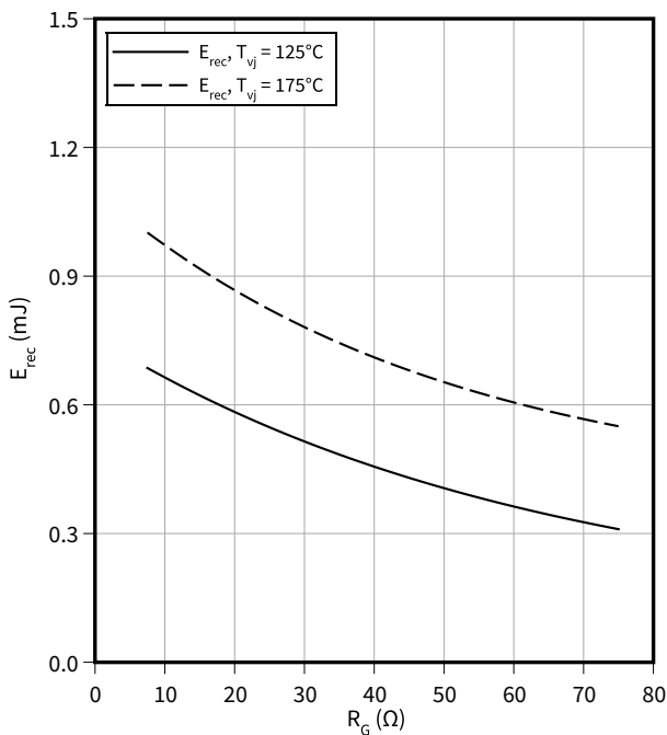
スイッチング損失 (typical), Diode、インバータ E_{rec} = f(R_G) I_F = 15 \text{ A} , V_{CC} = 600 \text{ V}
