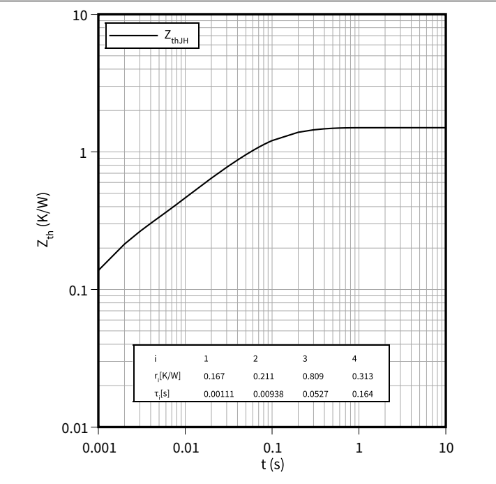
瞬态热阻抗, 二极管,整流器 Z_{th} = f(t)
