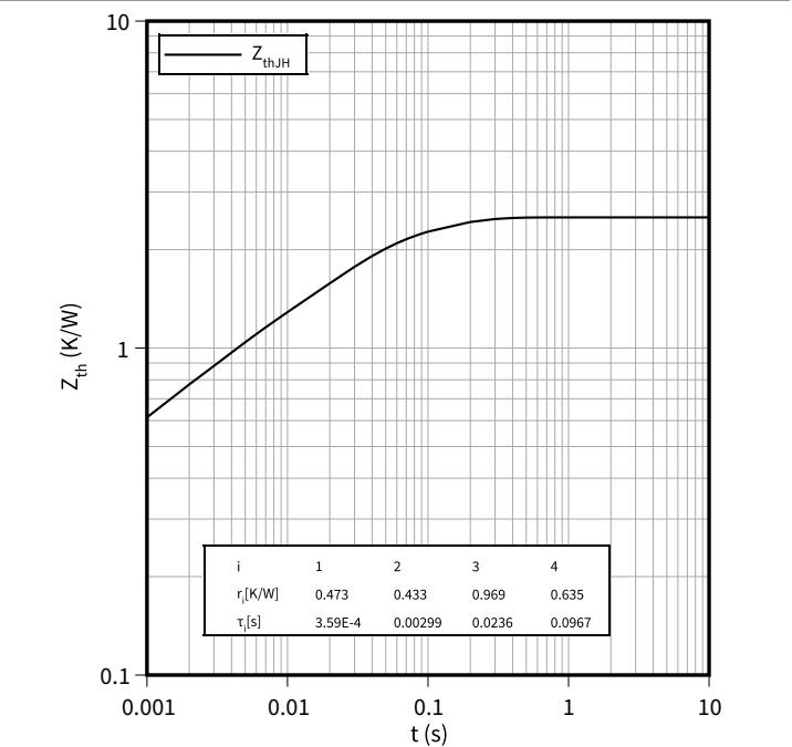
過渡熱インピーダンス, Diode、インバータ Z_{th} = f(t)
