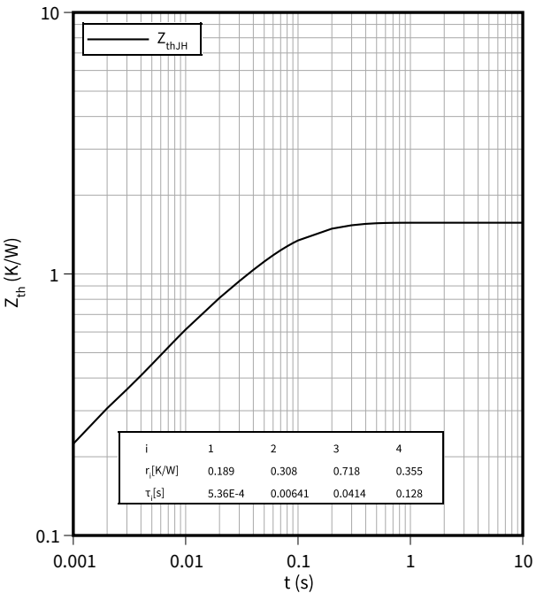
過渡熱インピーダンス, IGBT- インバータ Z_{th} = f(t)
