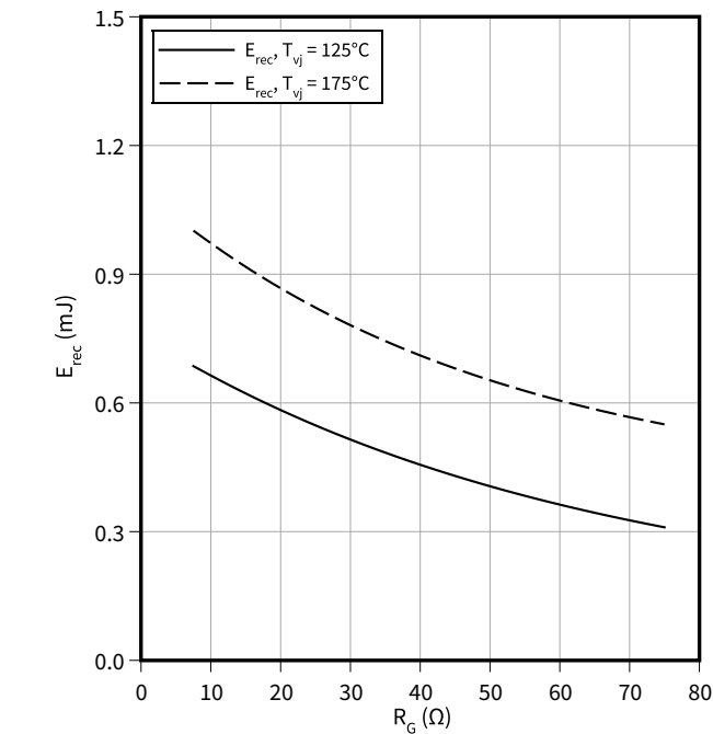
开关损耗（典型），二极管,逆变器 E_{rec} = f(R_G) I_F = 15 A, V_{CC} = 600 V
