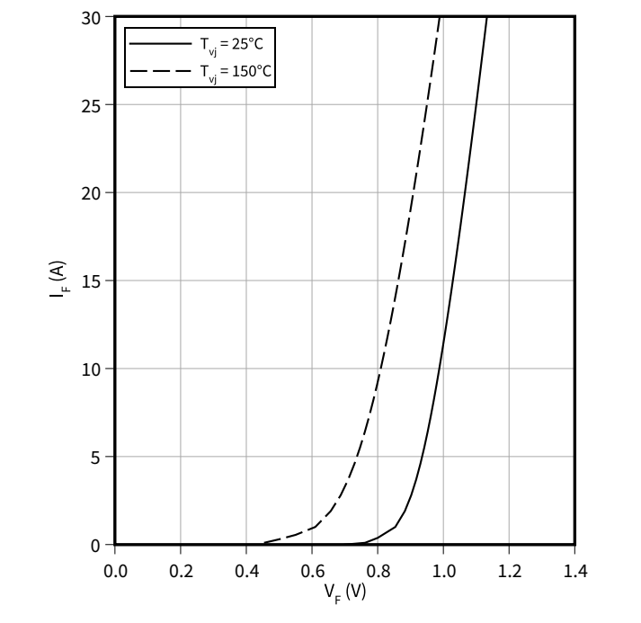
正向特性（典型), 二极管, 整流器
