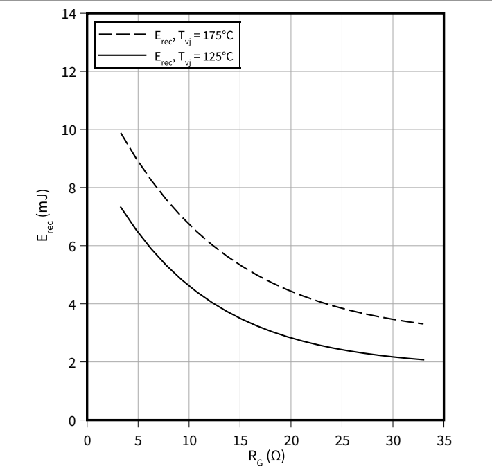
开关损耗（典型），二极管,逆变器 E_{rec} = f(R_G) I_F = 150 A, V_{CC} = 600 V
