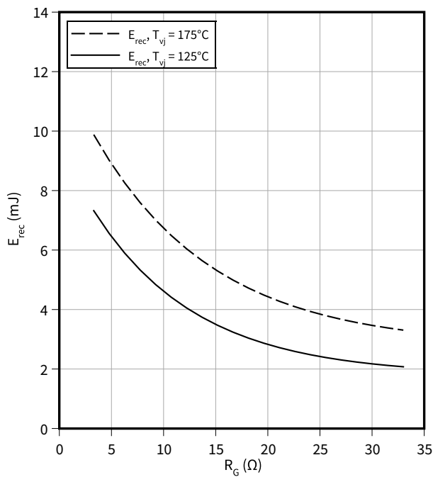
スイッチング損失 (typical), Diode、インバータ E_{rec} = f(R_G) V_{CE} = 600\ \text{V} , I_F = 150\ \text{A}
