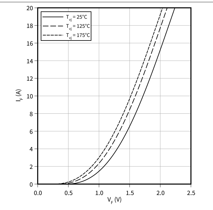
順電圧特性 (typical), Diode、ブレーキチョッパ I_F = f(V_F)
