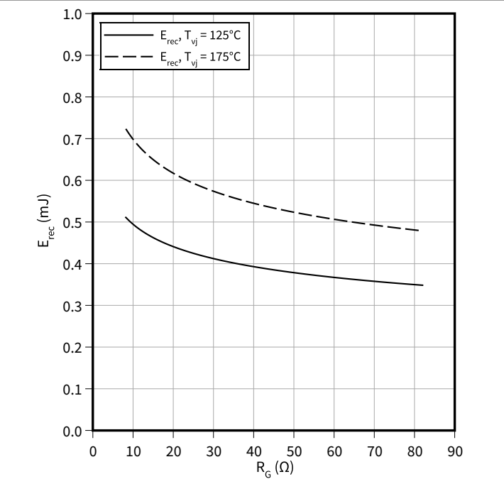
スイッチング損失 (typical), Diode、インバータ E_{rec} = f(R_G) I_F = 10\ \text{A} , V_{CC} = 600\ \text{V}
