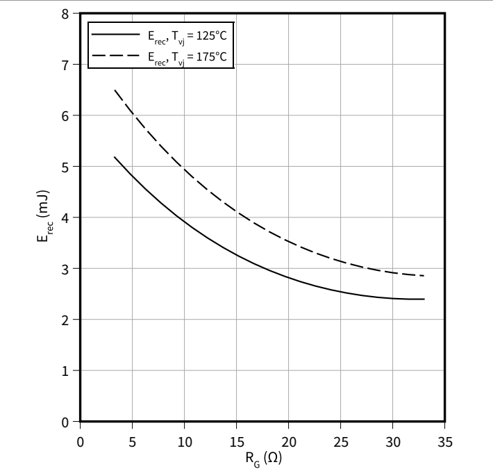
开关损耗（典型），二极管，逆变器 E_{rec} = f(R_G) I_F = 100\text{ A}, V_{CC} = 600\text{ V}
