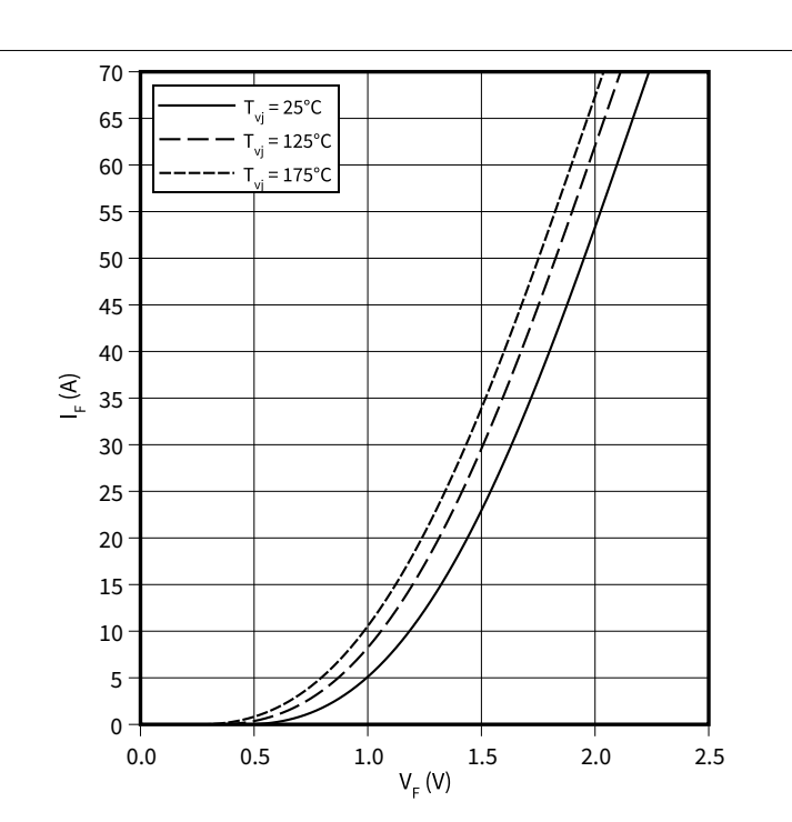
正向偏压特性（典型), 二极管, 制动-斩波器 I_F = f(V_F)
