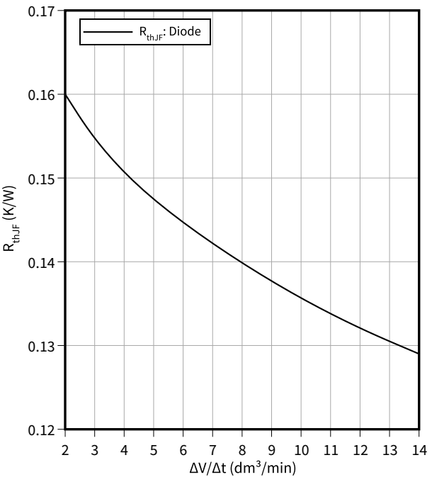
热阻抗, 二极管, 逆变器
