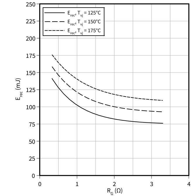
开关损耗（典型），二极管,逆变器 E_{rec} = f(R_G) I_F = 900\ \text{A} , V_{CC} = 900\ \text{V}
