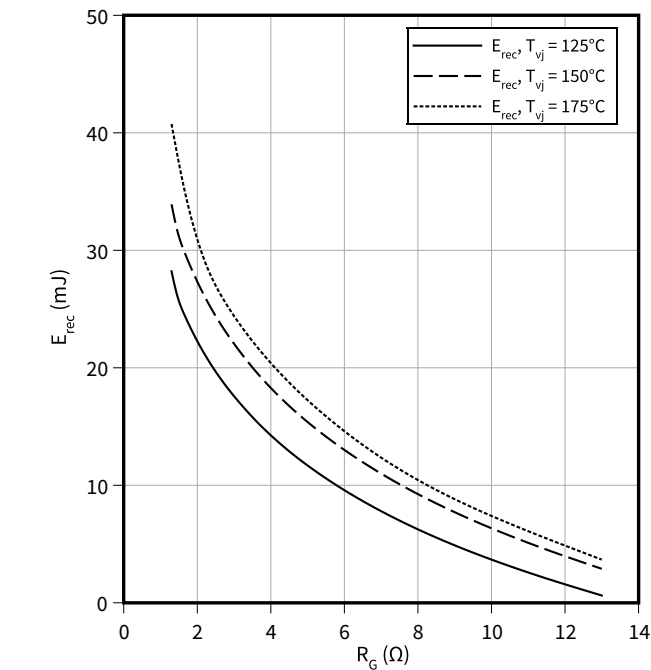
开关损耗（典型），二极管,逆变器 E_{rec} = f(R_G) V_{CE} = 600 V, I_F = 1000 A
