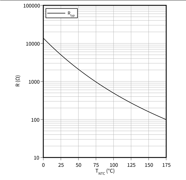
温度特性, 负温度系数热敏电阻 R = f(T_{\text{NTC}})
