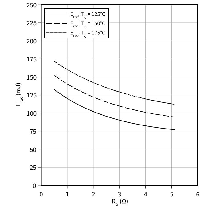
开关损耗（典型），二极管,逆变器 E_{rec} = f(R_G) I_F = 750 A, V_{CC} = 900 V
