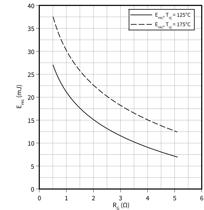
开关损耗（典型），二极管，逆变器 E_{rec} = f(R_G) I_F = 750\ \text{A} , V_{CC} = 600\ \text{V}
