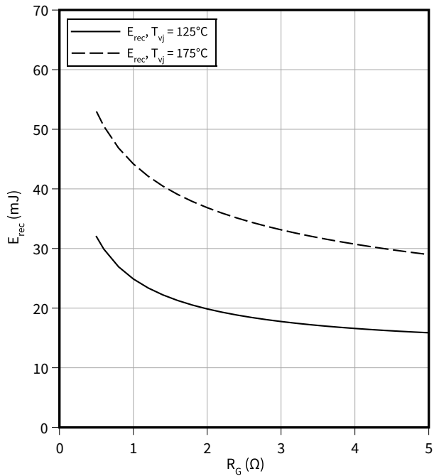
スイッチング損失 (typical), Diode、インバータ E_{rec} = f(R_G) I_F = 750\text{ A} , V_{CC} = 600\text{ V}
