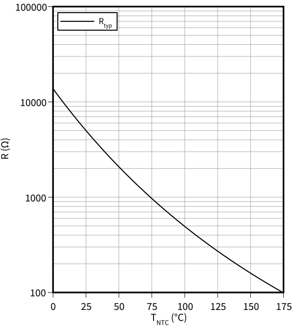
サーミスタの温度特性, NTC-サーミスタ R = f(T_{NTC})
