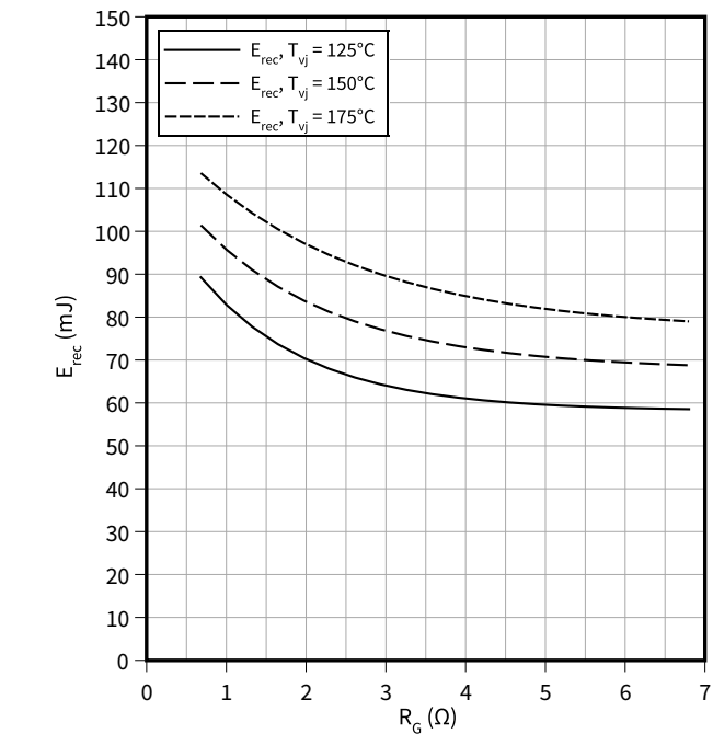
开关损耗（典型），二极管,逆变器 E_{rec} = f(R_G) I_F = 600 A , V_{CC} = 900 V
