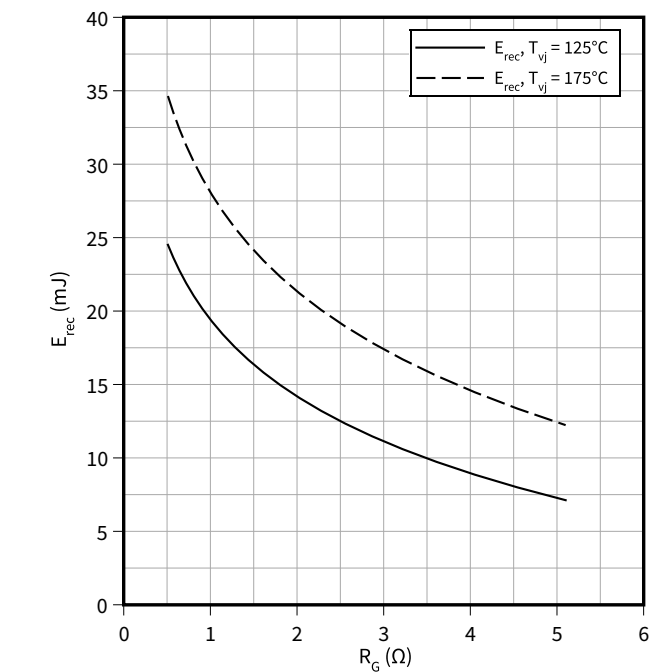
开关损耗（典型），二极管，逆变器 E_{rec} = f(R_G) I_F = 600 A, V_{CC} = 600 V
