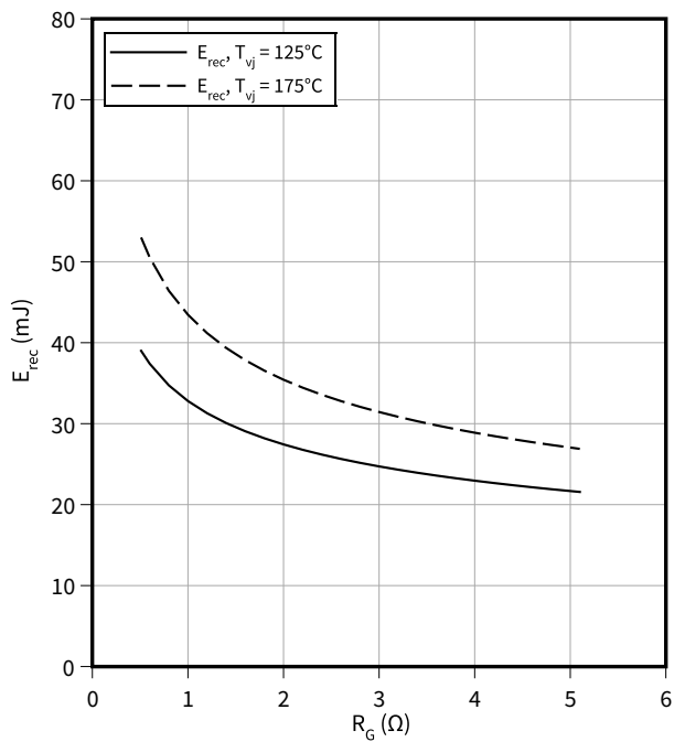
スイッチング損失 (typical), Diode、インバータ E_{rec} = f(R_G) I_F = 600 \text{ A} , V_{CC} = 600 \text{ V}
