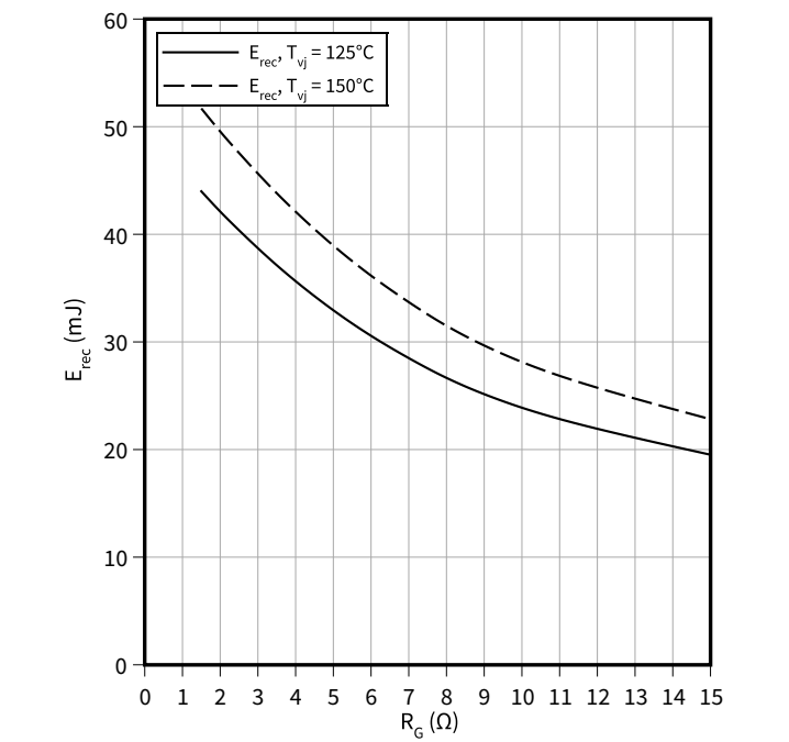
开关损耗（典型），二极管，逆变器 E_{rec} = f(R_G) I_F = 600\ \text{A} , V_{CC} = 600\ \text{V}
