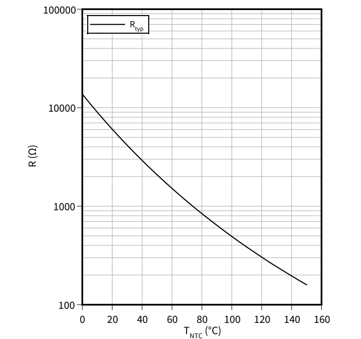
温度特性, 负温度系数热敏电阻
