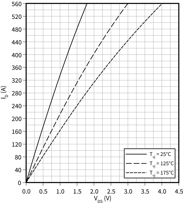
输出特性 (典型), MOSFET
