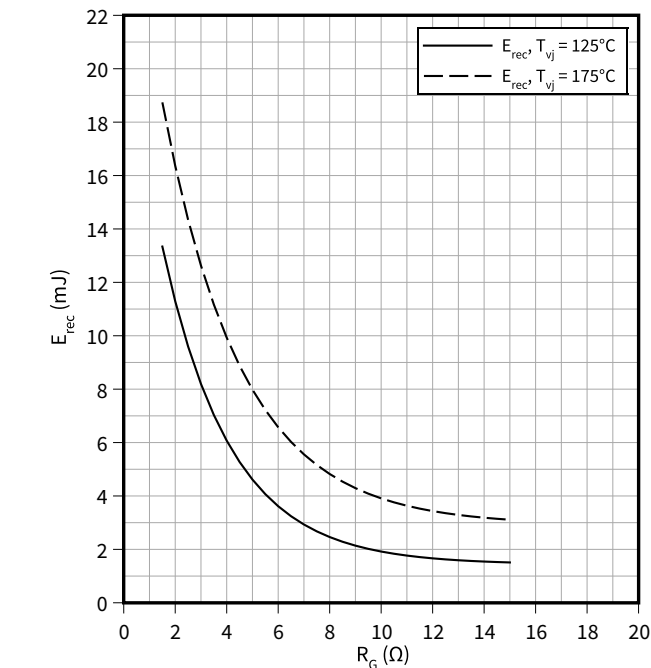
开关损耗（典型），二极管,逆变器 E_{rec} = f(R_G) I_F = 300 A, V_{CC} = 600 V
