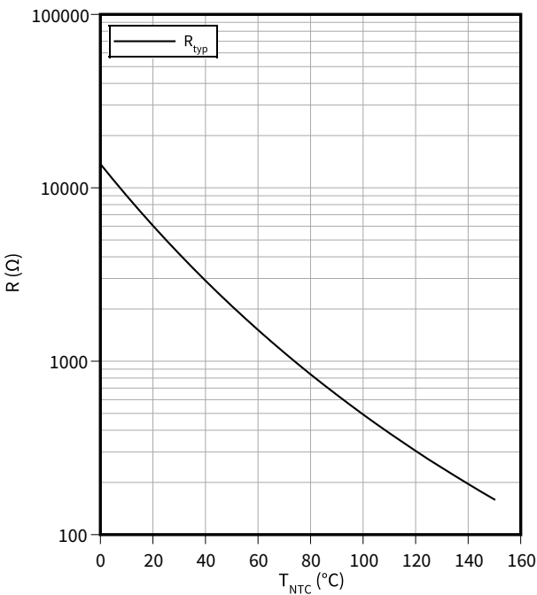
温度特性，负温度系数热敏电阻
