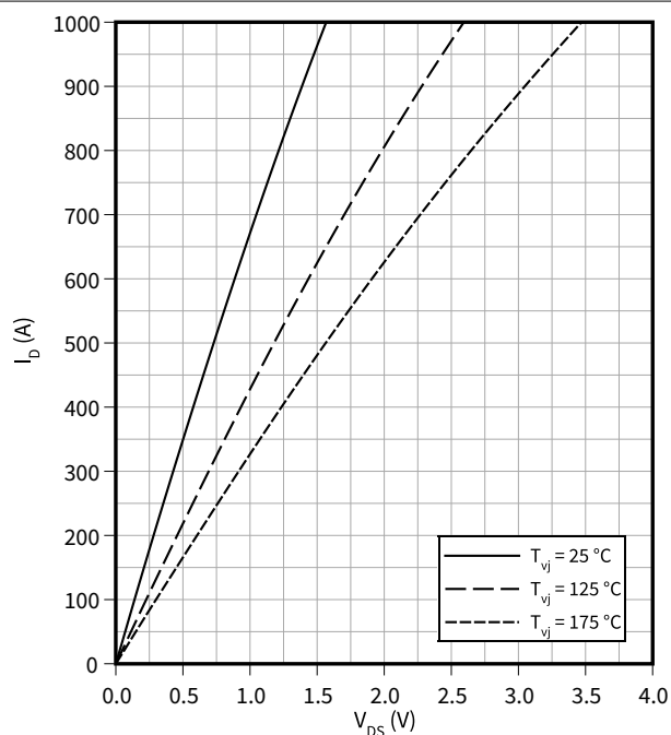
出力特性 (typical), MOSFET, T1 / T2
