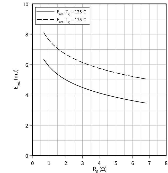
开关损耗（典型），二极管,逆变器 E_{rec} = f(R_G) I_F = 100 \text{ A} , V_{CC} = 600 \text{ V}
