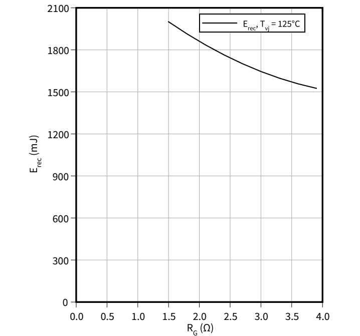
开关损耗（典型), 二極體, 反轉 E_{rec} = f(R_G) V_{CE} = 3600\text{ V} , I_F = 500\text{ A}
