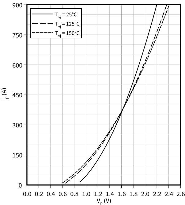
正向特性（典型）, 二极管, 制动-斩波器 I_F = f(V_F)
