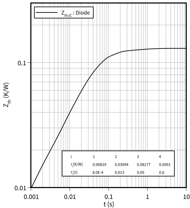
瞬态热阻抗, 二極體, 反轉 Z_{th} = f(t)
