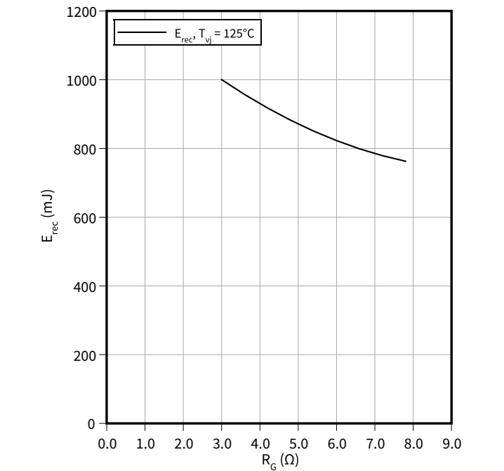
开关损耗（典型), 二极管，制动-斩波器 E_{rec} = f(R_G) V_{CE} = 3600\text{ V} , I_F = 250\text{ A}
