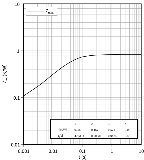
過渡熱インピーダンス, Diode, D11 / D12 / D21 / D22
