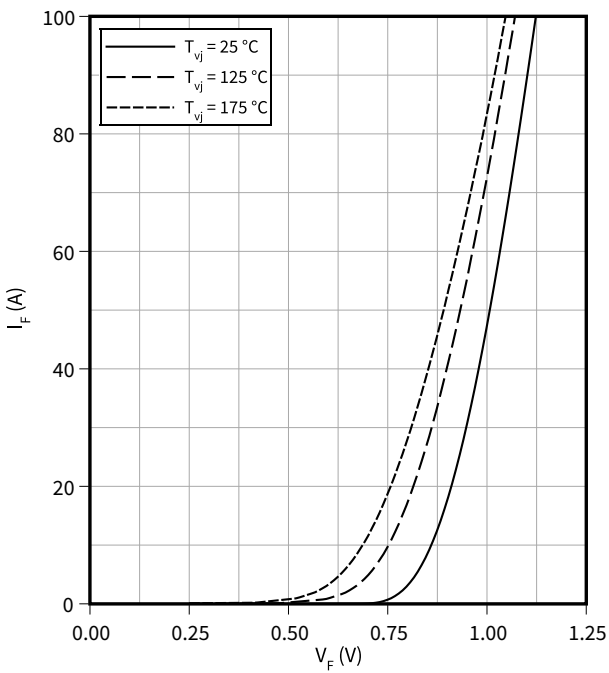
順電圧特性 (typical), Diode, D13 / D14 / D23 / D24
