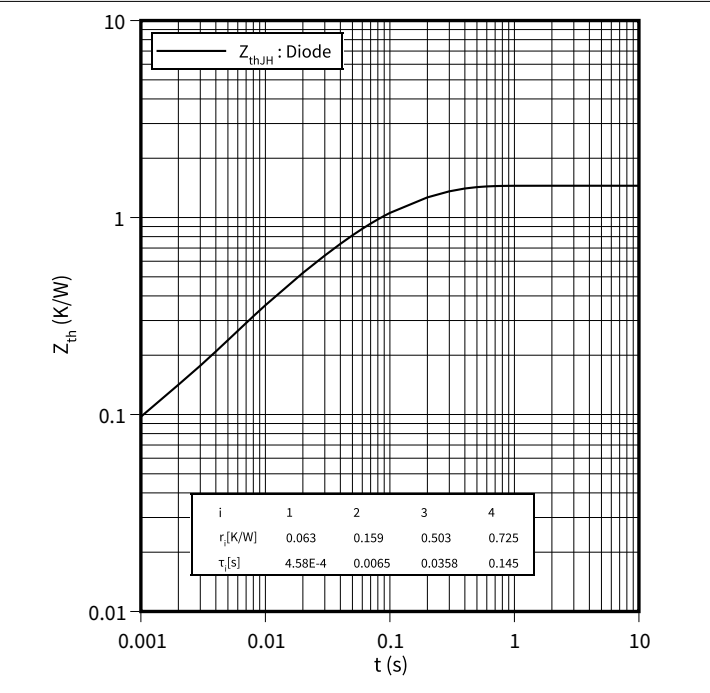
瞬态热阻抗, 二极管, 整流器
