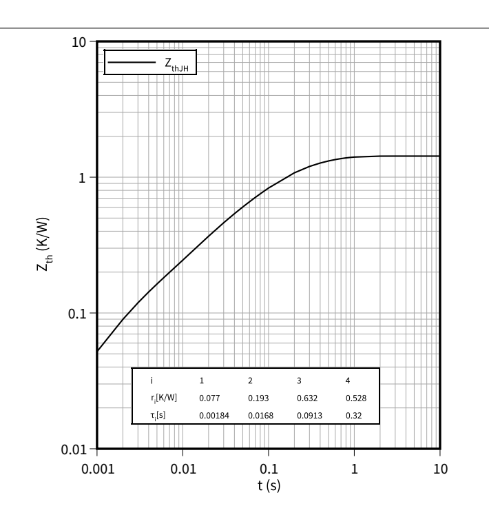
瞬态热阻抗, 二极管, 整流器
