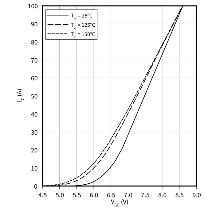
伝達特性 (typical) , IGBT, ブースト I_C = f(V_{GE}) V_{CE} = 20\text{ V}
