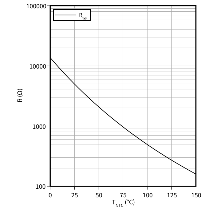
サーミスタの温度特性, NTC-サーミスタ R = f(T_{NTC})
