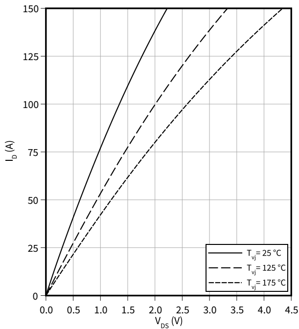
Ausgangskennlinienfeld (typisch), MOSFET, T1-T4
