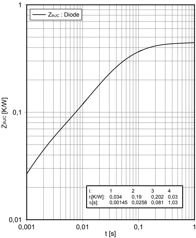
過渡熱インピーダンス Diode、インバータ transient thermal impedance Diode, Inverter Z_{thJC} = f(t)
