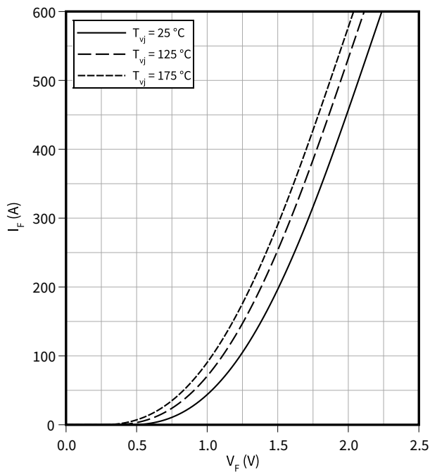
順電圧特性 (typical), ダイオード、D5 / D6
