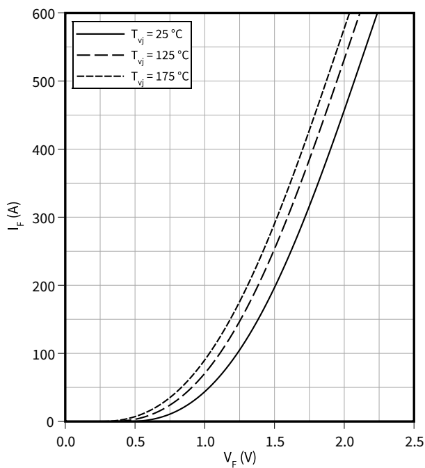
正向特性（典型），二极管，D5 / D6
